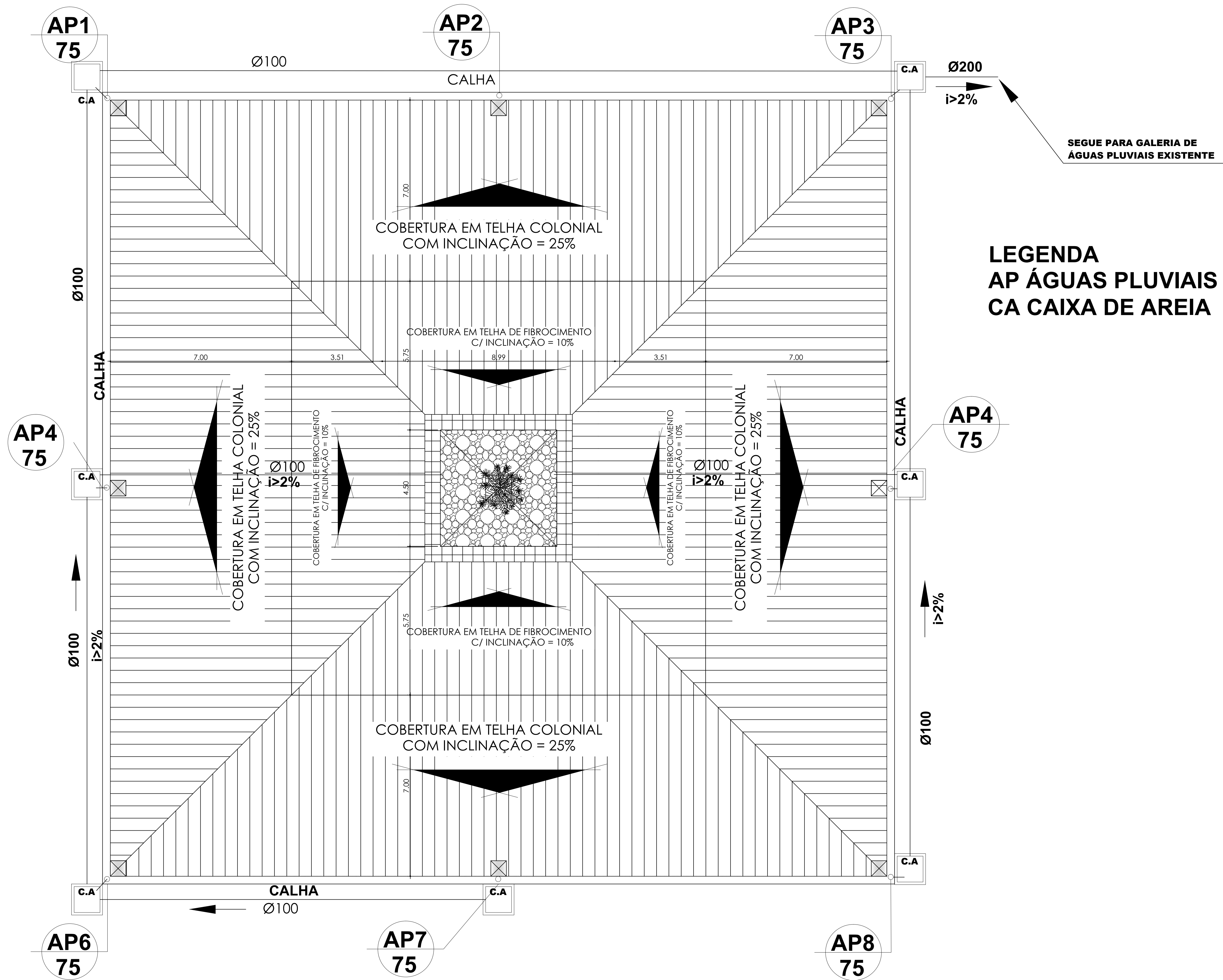
PROJETO DE DRENAGEM ESCALA 1/75
