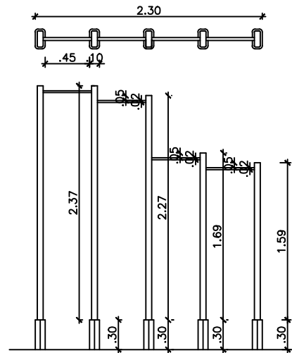
EQ. 01 BARRA PARA FLAXÃO DE BRAÇOS VERTICAL 1/50
