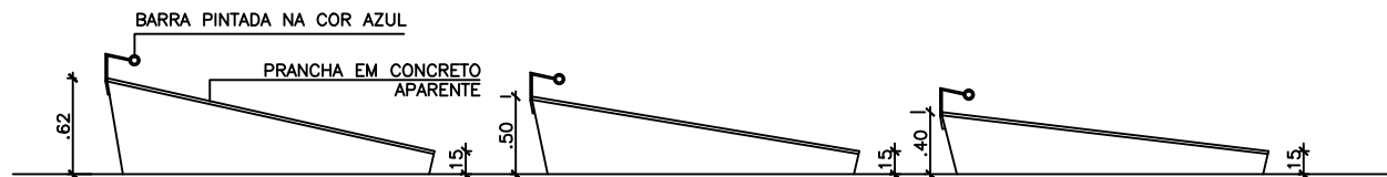
EQ. 02 PRANCHAS DE EXERCÍCIO ABDOMINAIS ESC - 1/50
