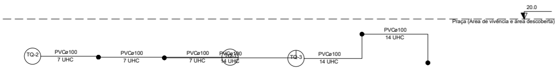
Esquema vertical sanitário Escala: 1:50
