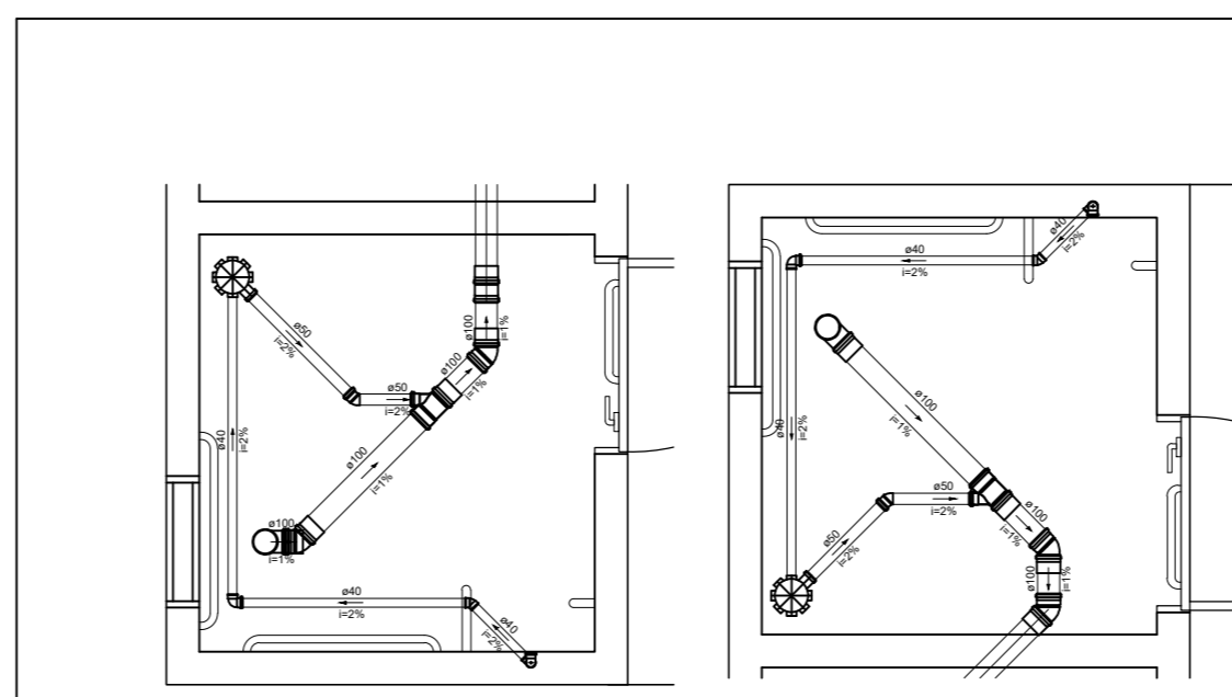
Detalhe S2 Escala 1:25
