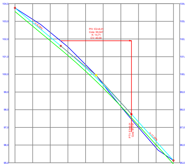
RUA DANIEL DINIZ - E0+0 ATÉ E4+9,84 PERFIL LONGITUDINAL - ESC.: V=1:50 H=1:500
