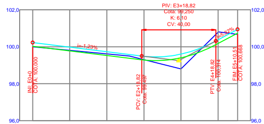
RUA JOSÉ MARIA GONÇALVES VALE - E0+0 ATÉ E5+10,51 PERFIL LONGITUDINAL - ESC.: V=1:100 H=1:1000
