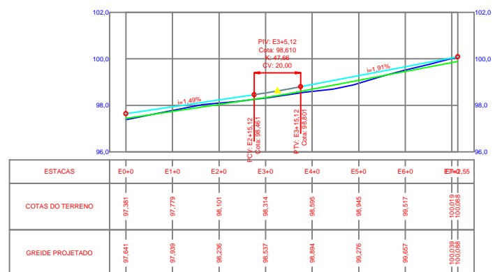
RUA JULIA TEIXEIRA - E0+0 ATÉ E7+2,55 PERFIL LONGITUDINAL - ESC.: V=1:100 H=1:1000
