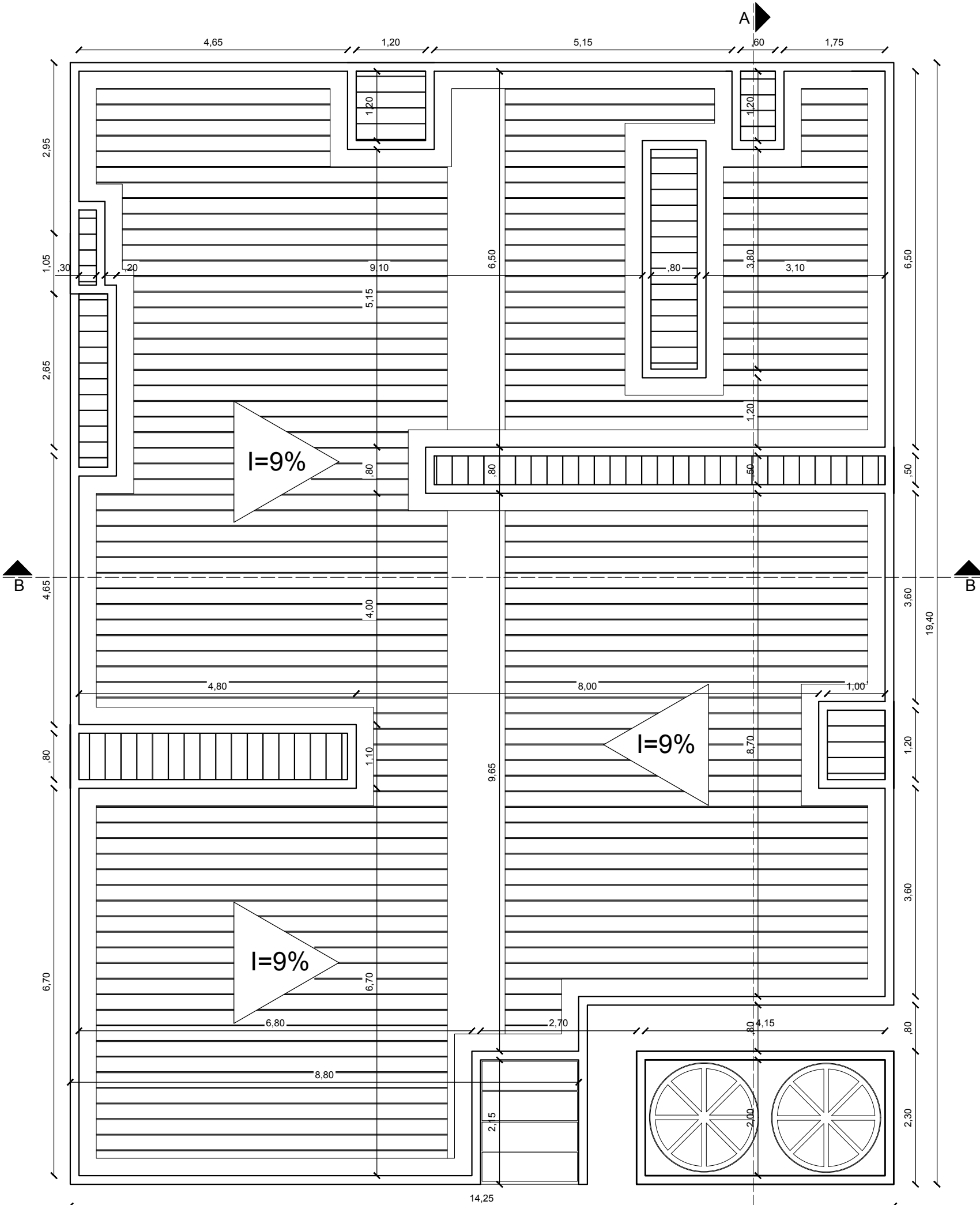
PLANTA COBERTURA ESC.: 1/75
