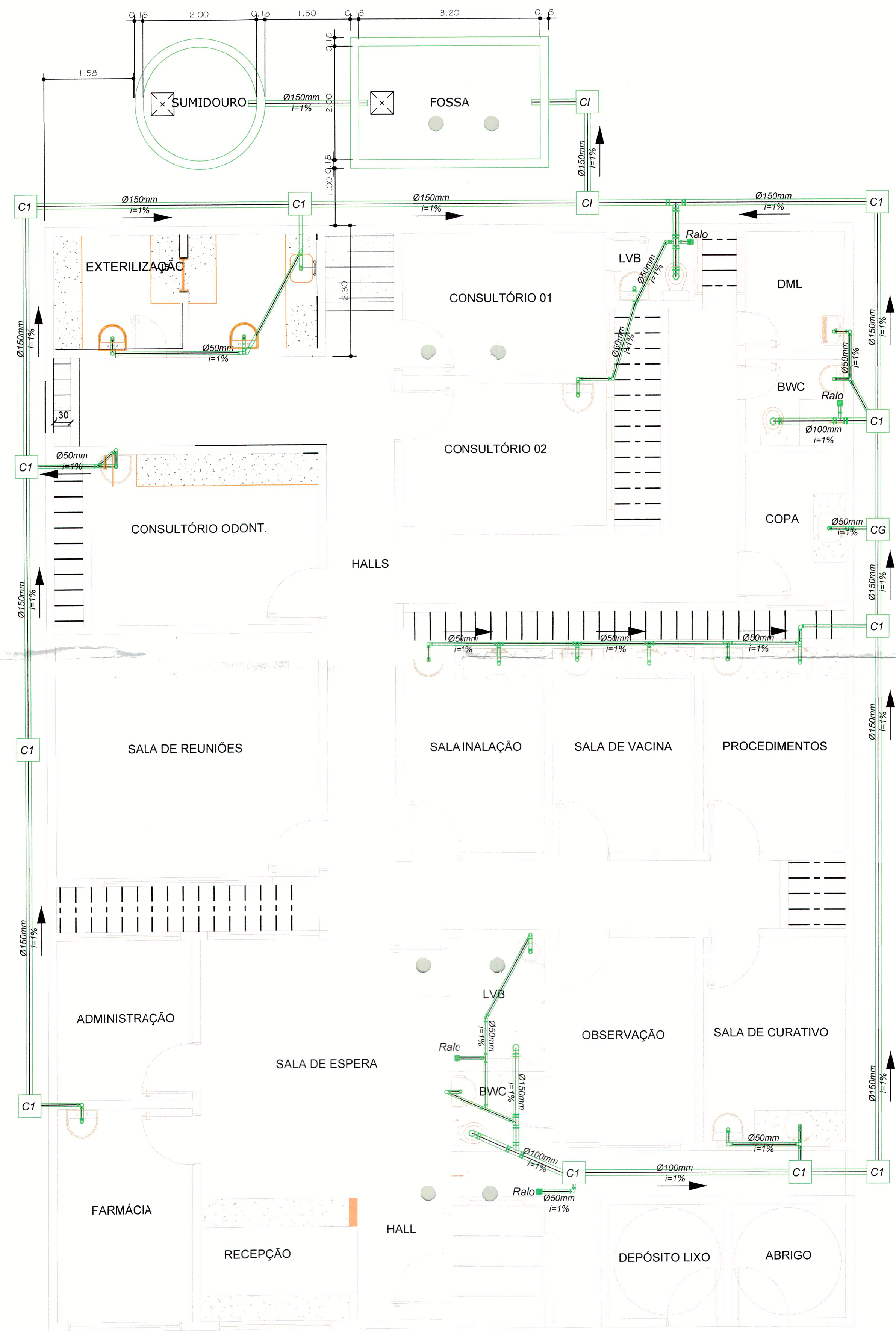
PLANTA BAIXA DO POSTO DE SAÚDE. Escala: 1/50
